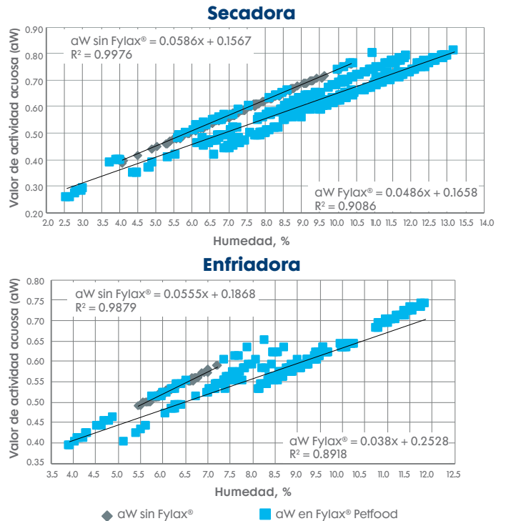
Figura 2: Evaluación del líquido Fylax® Petfood en la secadora y la enfriadora de una planta elaboradora de alimentos para mascotas en Latinoamérica.
